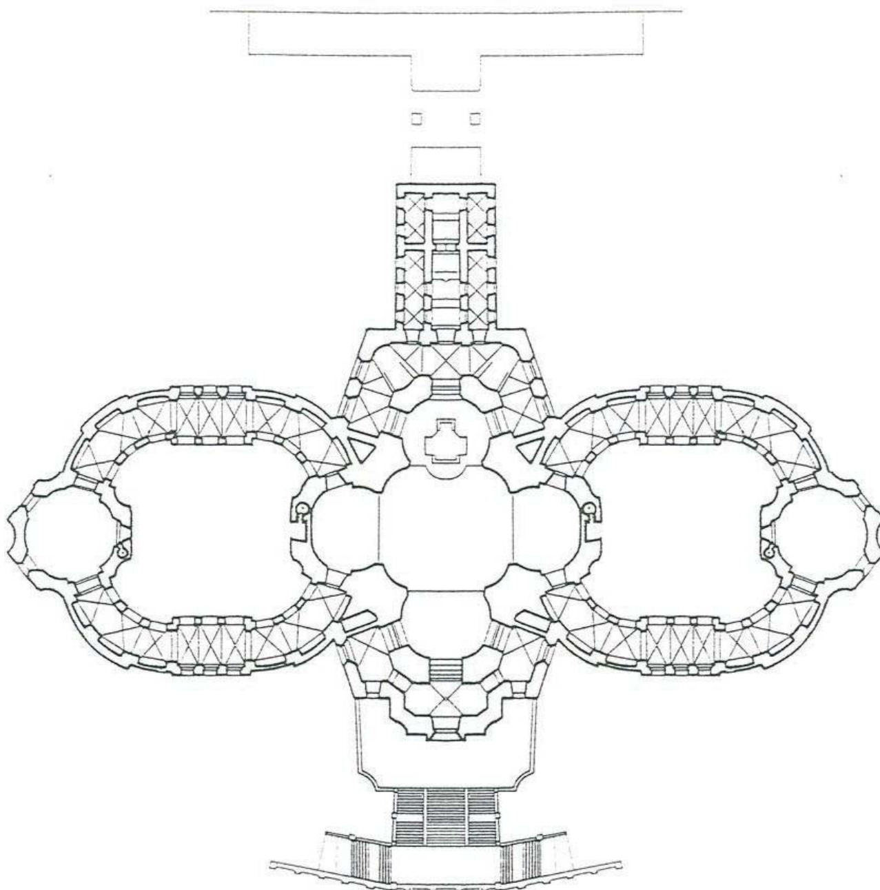
Projekt půdorysu kostela s původním plánem dvou ambitů
